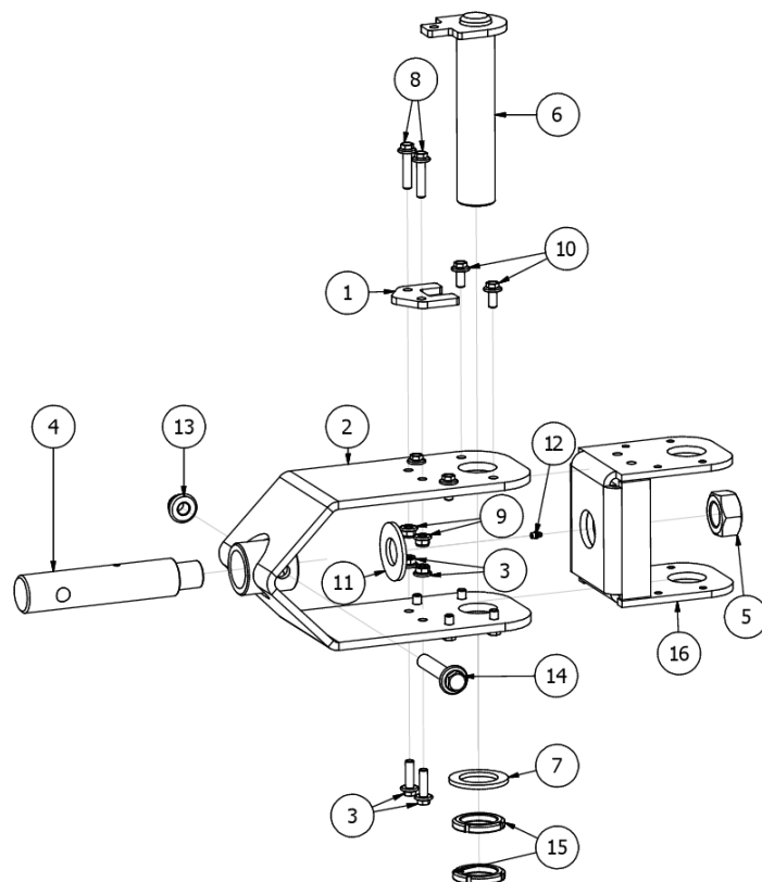
Rys. 8 BT00821-S Głowica zaczepu - skręcana
