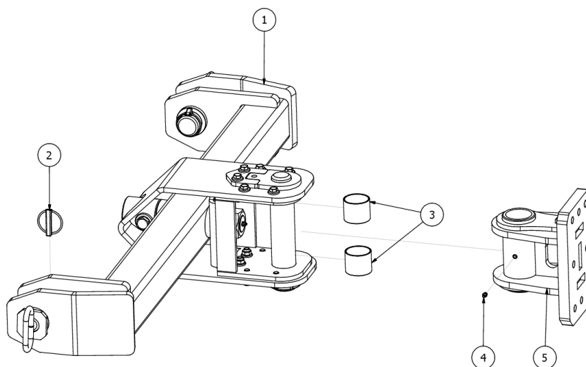
Rys. 6 AU01385-02 wahliwy kat. 2+3 Typ "U"
