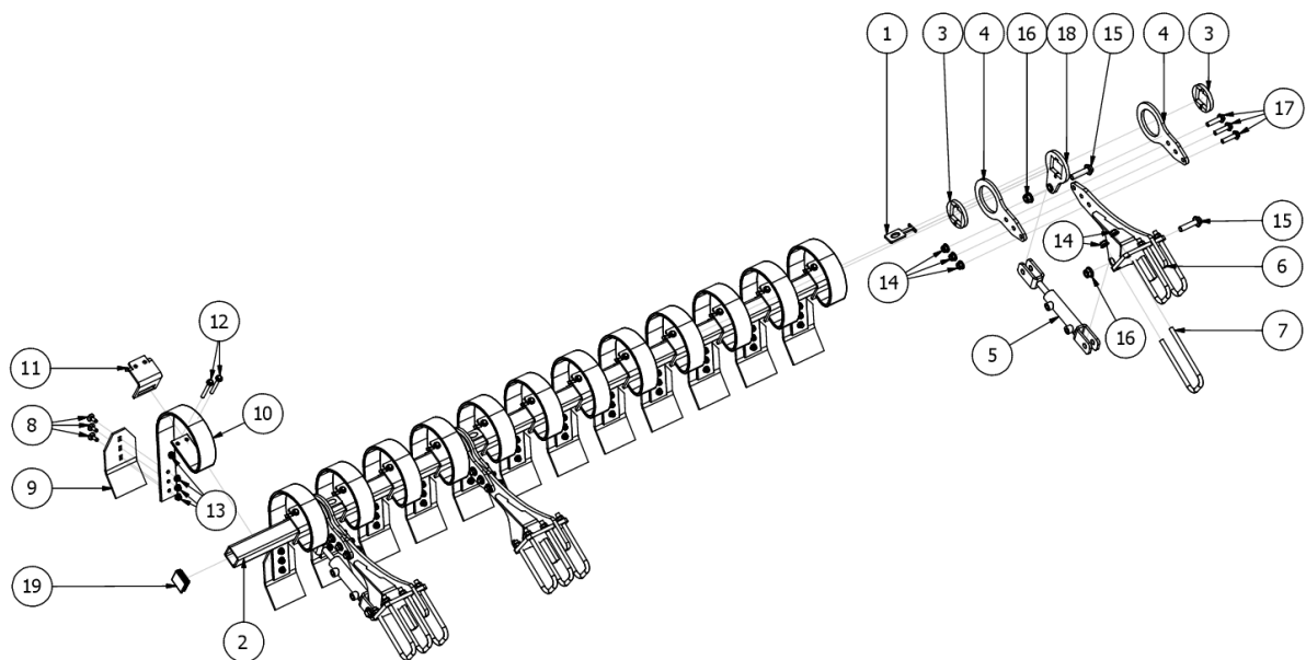
Rys. 24 AU02163 Włoka środkowa
