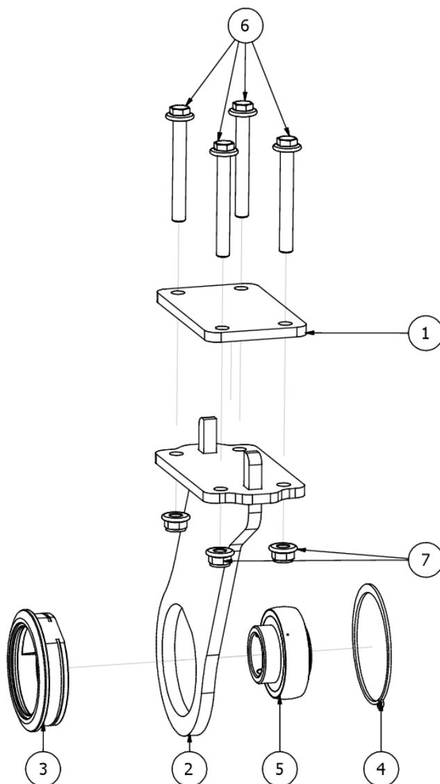
Rys. 20 AU02405 Uchwyt pod wał Cambridge Hestile 82 lewy
