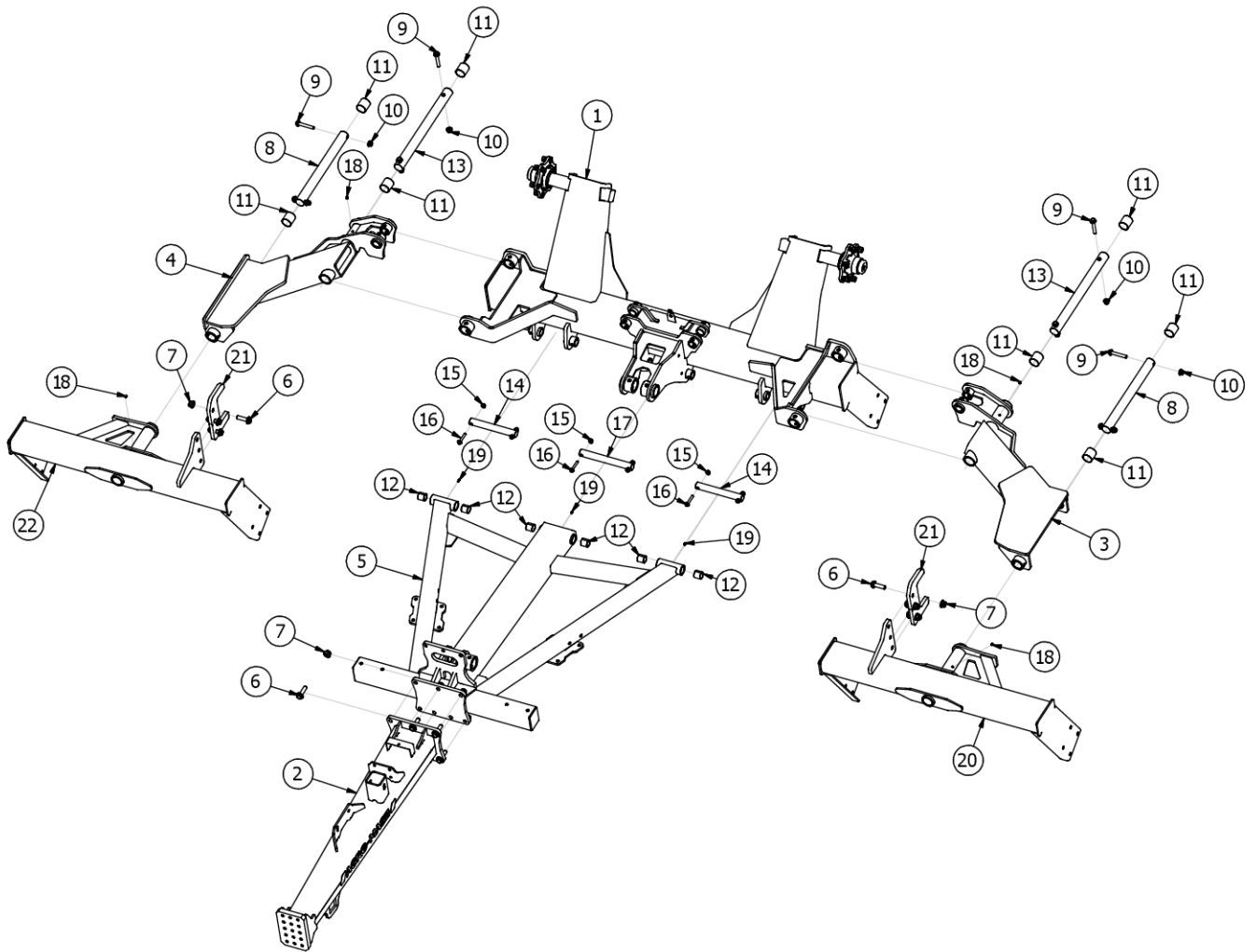
Rys. 2 AU02362 Rama Kompletna Hestile 45
