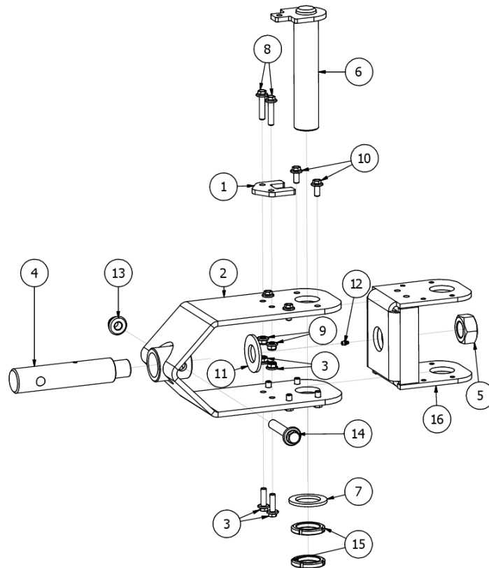
Rys. 9 BT00821-S Głowica zaczepu - skręcana
