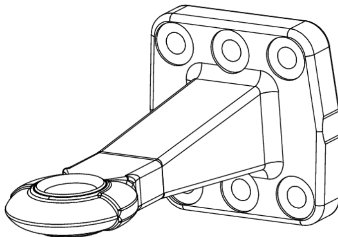
Rys. 5 RO00093 Zaczep oczkowy Fi40
