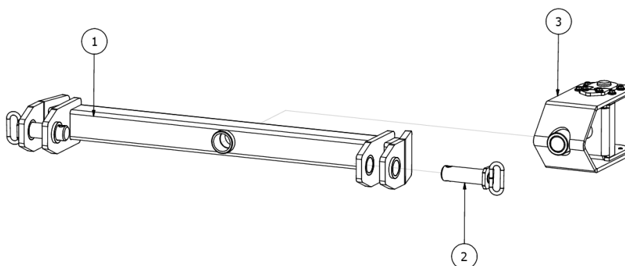
Rys. 8 BT02674-03 Zaczepek kat. 2 i 3
