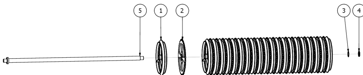
Rys. 17 AU01119 Wał Posiewny Fi 600
