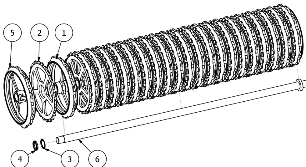
Rys. 15 EW01782 Wał Cambridge
