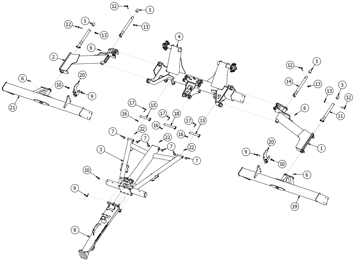
Rys. 2 AU02365 Kompletna Rama Hestile 63
