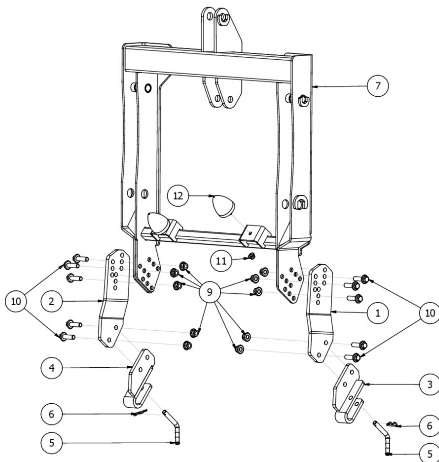
Rys. 10 AT00776 Hydropak Y regulowany
