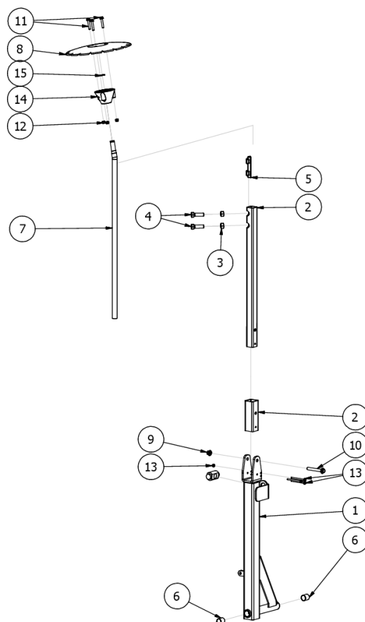
Rys. 27 SI04067 Znacznik lewy
