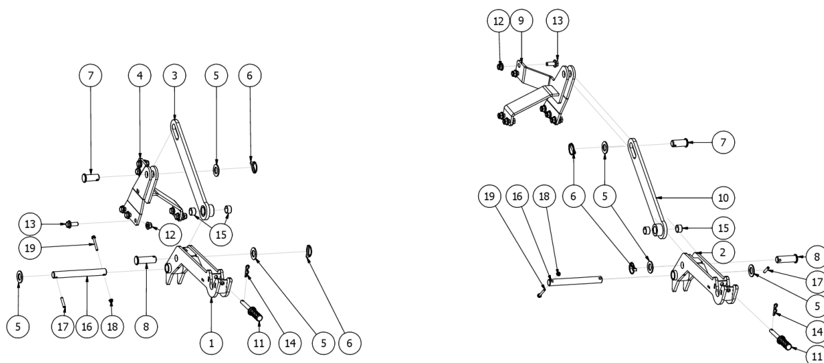
Rys. 11 AN00462 Sprzęg do połączenia z siewnikiem
