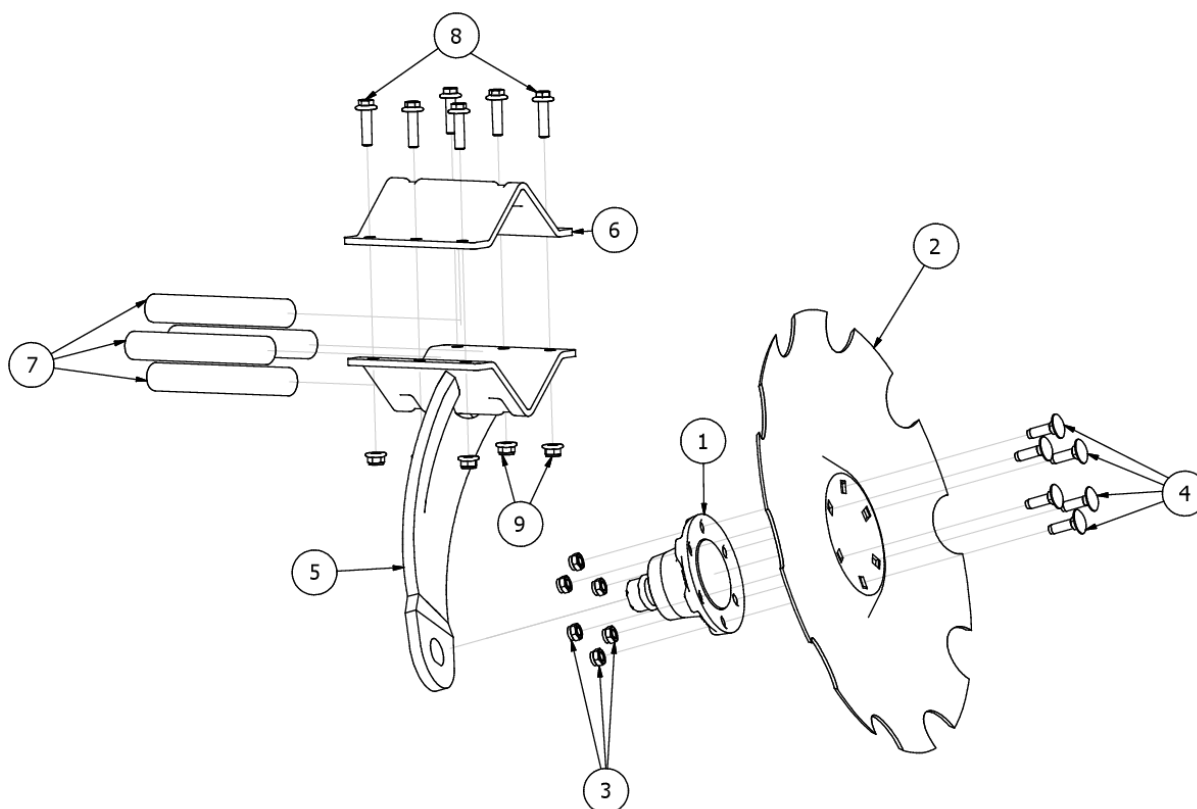
Rys. 15 EW02466M-02 Noga tłoczona prawa talerz P 560 skrajna szeroki daszek
