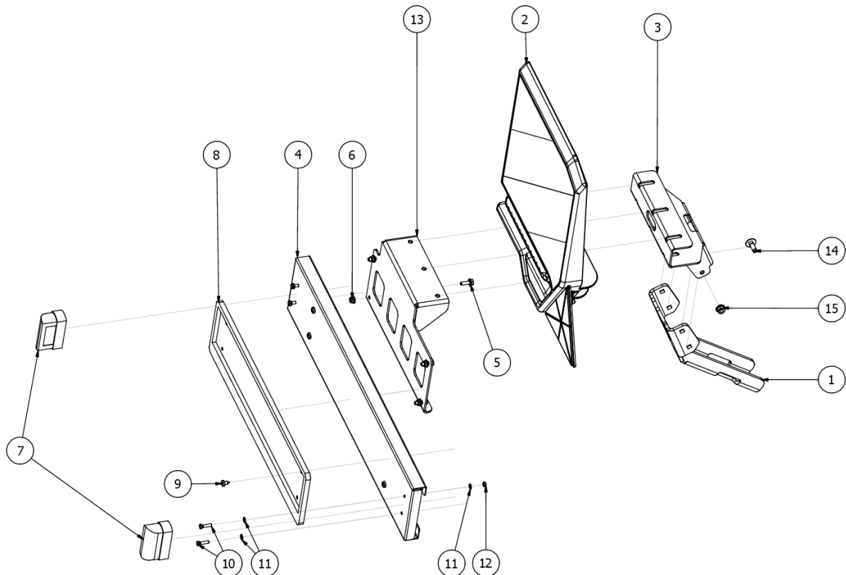
Rys. 37 AP03282 Oświetlenie tylne lewe
