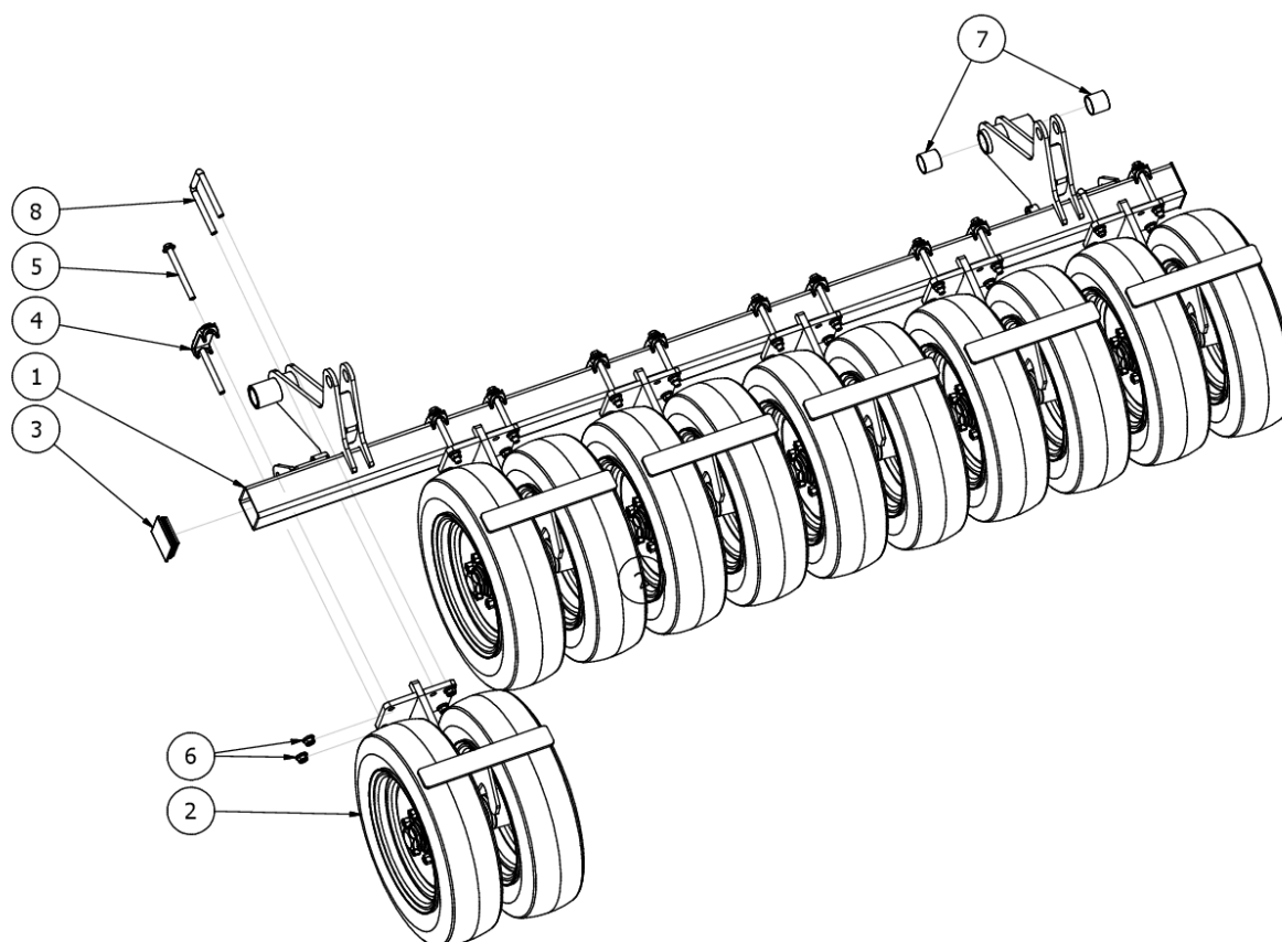
Rys. 12 AN00446 Wał oponowy
