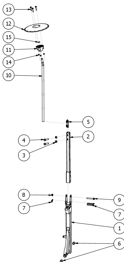
Rys. 28 SI04067M Znacznik prawy
