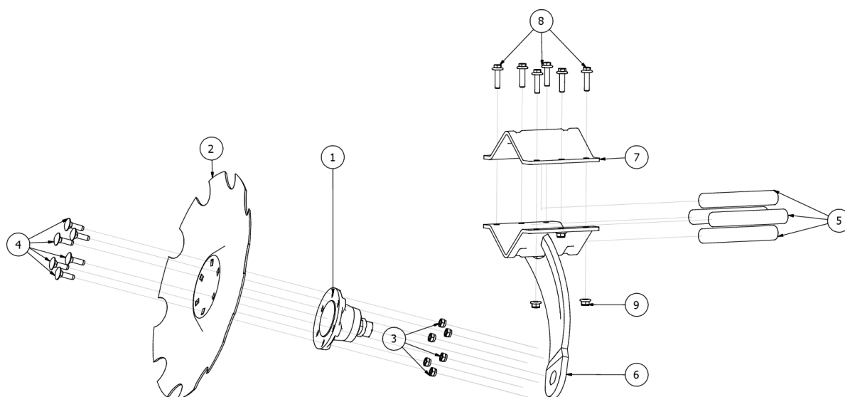
Rys. 14 EW02466-02 Noga tłoczona lewa talerz P 560 szeroki daszek
