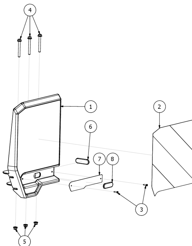
Rys. 32 EW03228 Tablica oświetlenia przednia prawa
