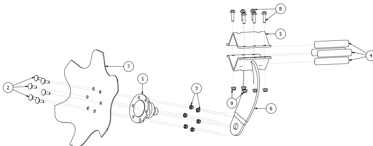
Rys. 23 EW02459M-06 Noga tłoczona prawa talerz C 510 skrajny wąski daszek
