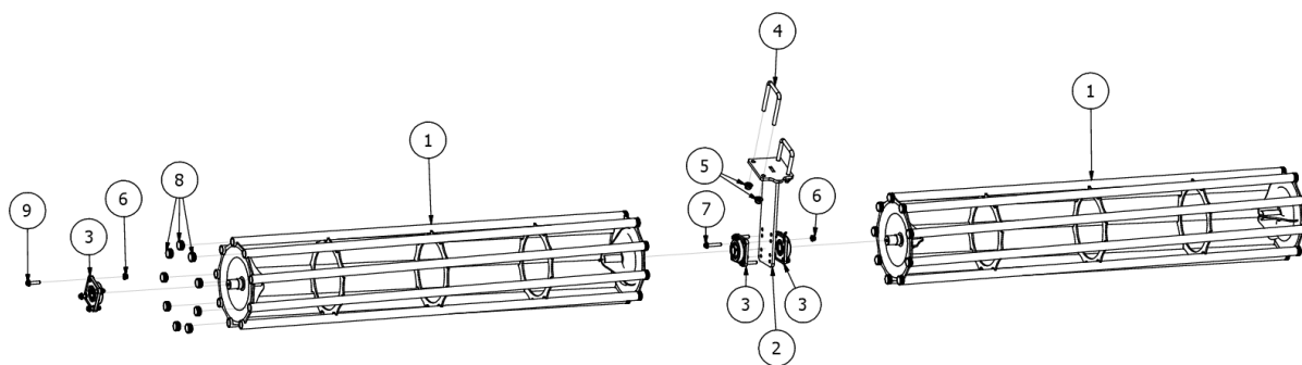
Rys. 7 AS00214 wał rurowy (śr. 400 mm)
