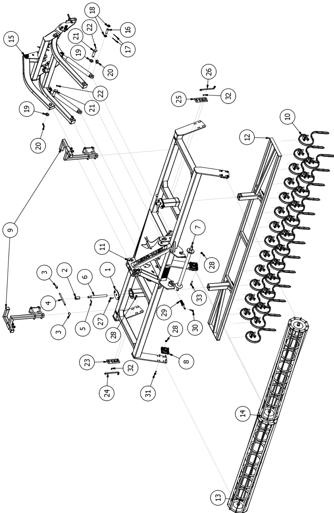
Rys. 1 A010R2 Agregat uprawowo-siewny dwa rzędy zębów 32x12mm
