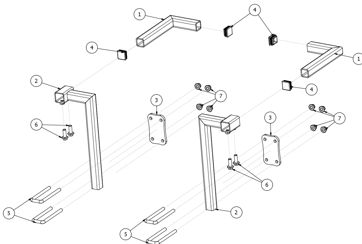
Rys. 4 AS00315 Komplet blokad kół siewnika
