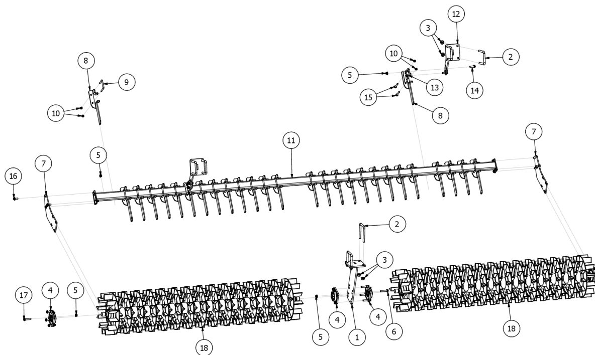
Rys. 9 AS00222 wał crossskill (śr. 400mm)
