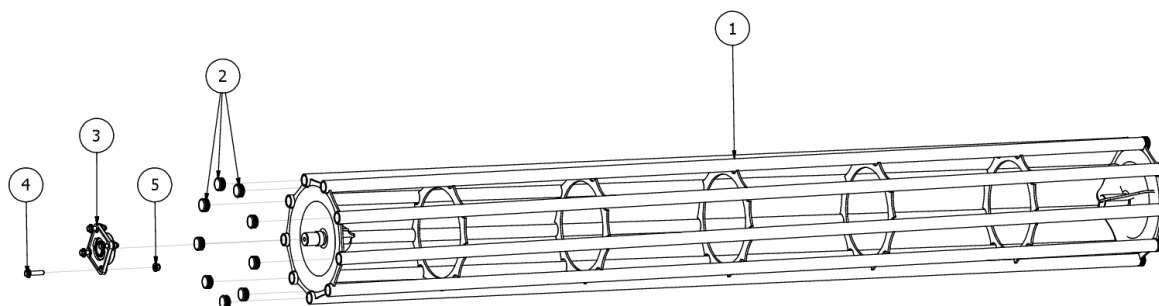
Rys. 7 AS00213 wał rurowy (śr. 400 mm)
