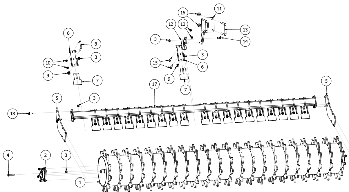
Rys. 8 AS00216 wał packer (śr. 400mm)
