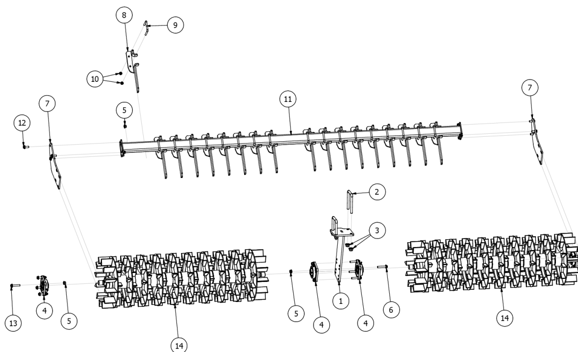
Rys. 9 AS00220 wał crossskill (śr. 400mm)
