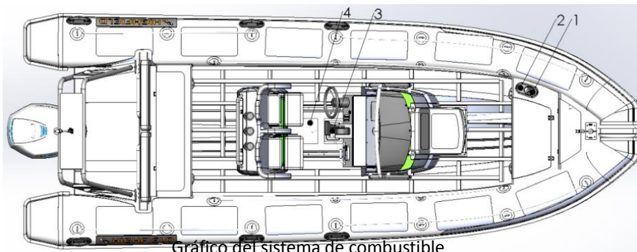
Gráfico del sistema de combustible
