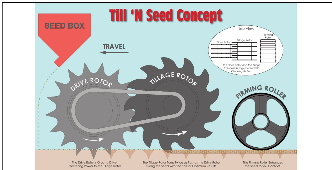
Figure 2-1: Till 'N Seed Concept
