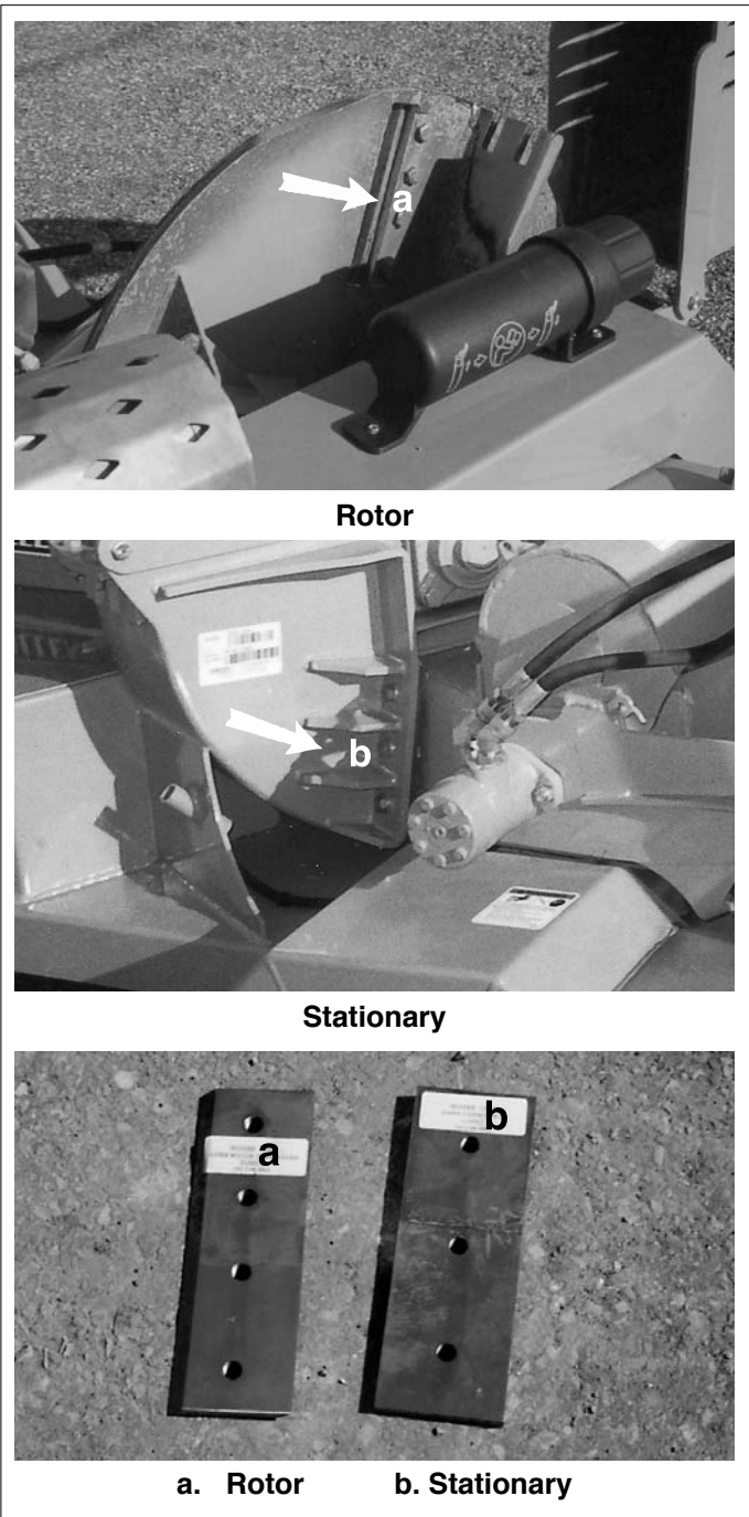
Fig. 22 BLADES
