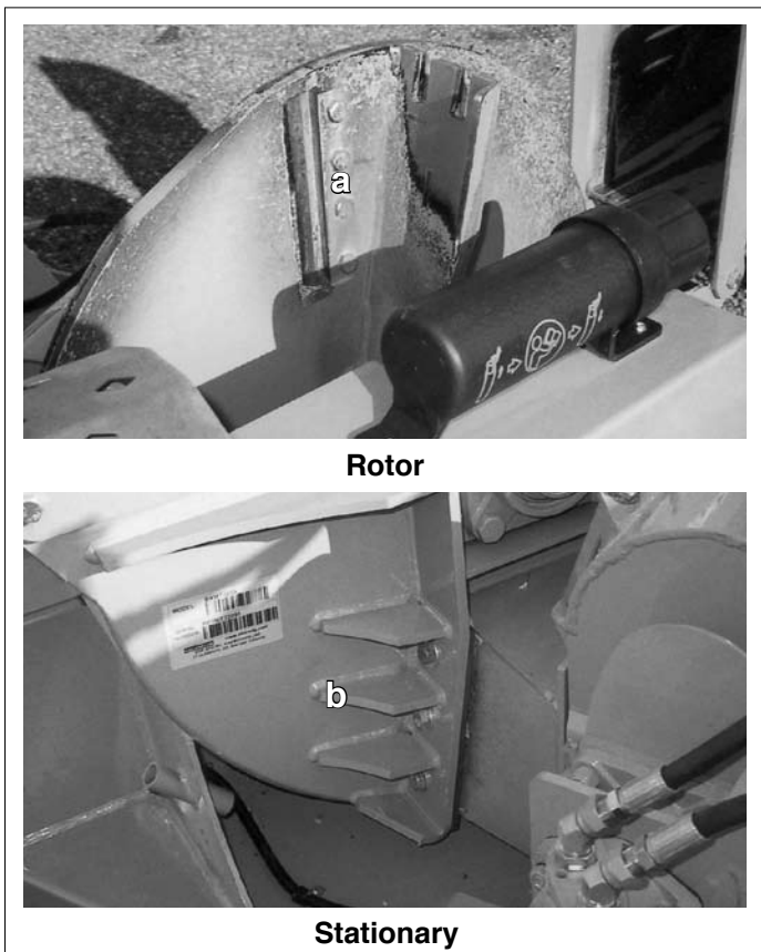
Fig. 35 BLADES
