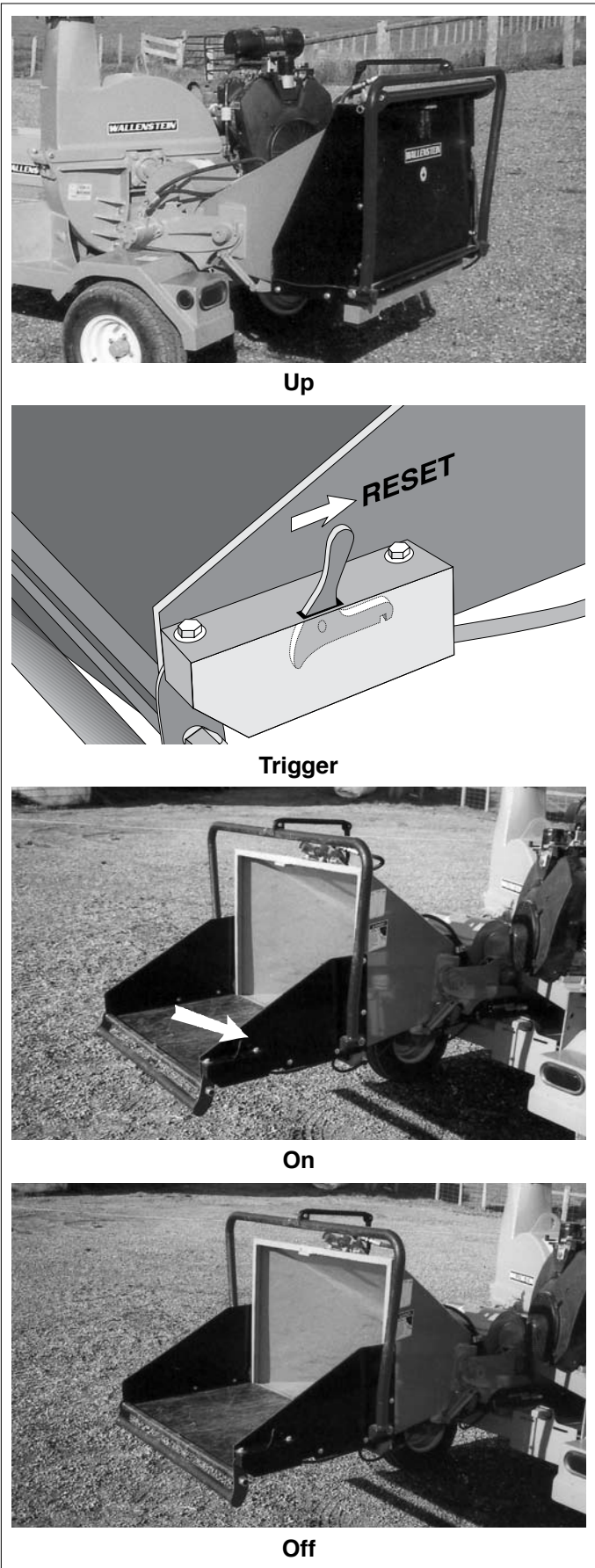
Fig. 25 PANIC BAR
